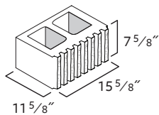
12x8x16 Stretcher
