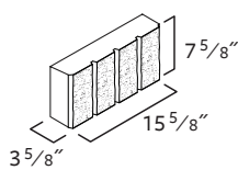
4x8x16 Solid
