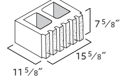
12x8x16 Stretcher
