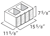
12x8x16 Stretcher
