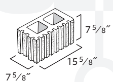
8x8x16 Return Corner
